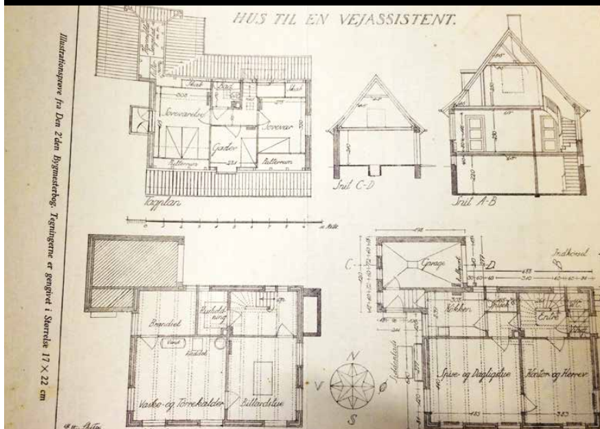
Eksempel på tegneøvelse for tømrerlærlinge fra den 2'nde Bygmesterbog fra 1934.
